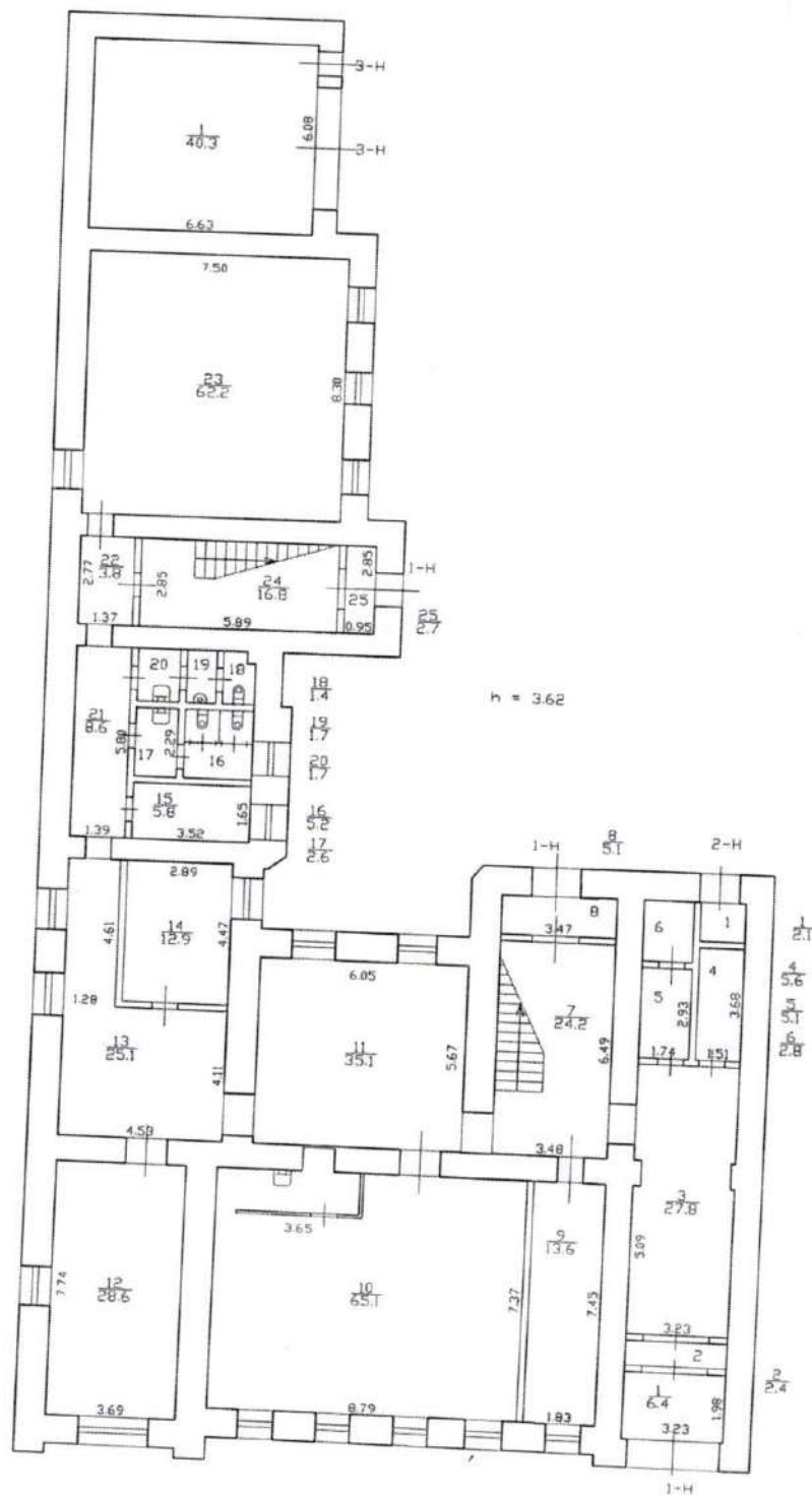
План 1 этажа.
